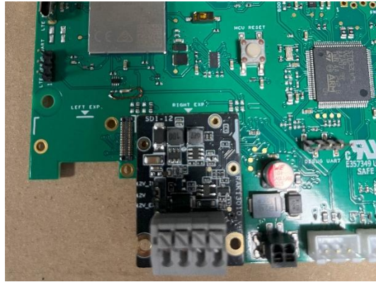
Figure 28: SDI12 Module
